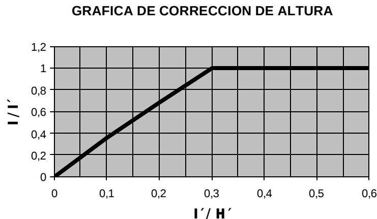
Gráfica 2. Corrección de la altura mínima
