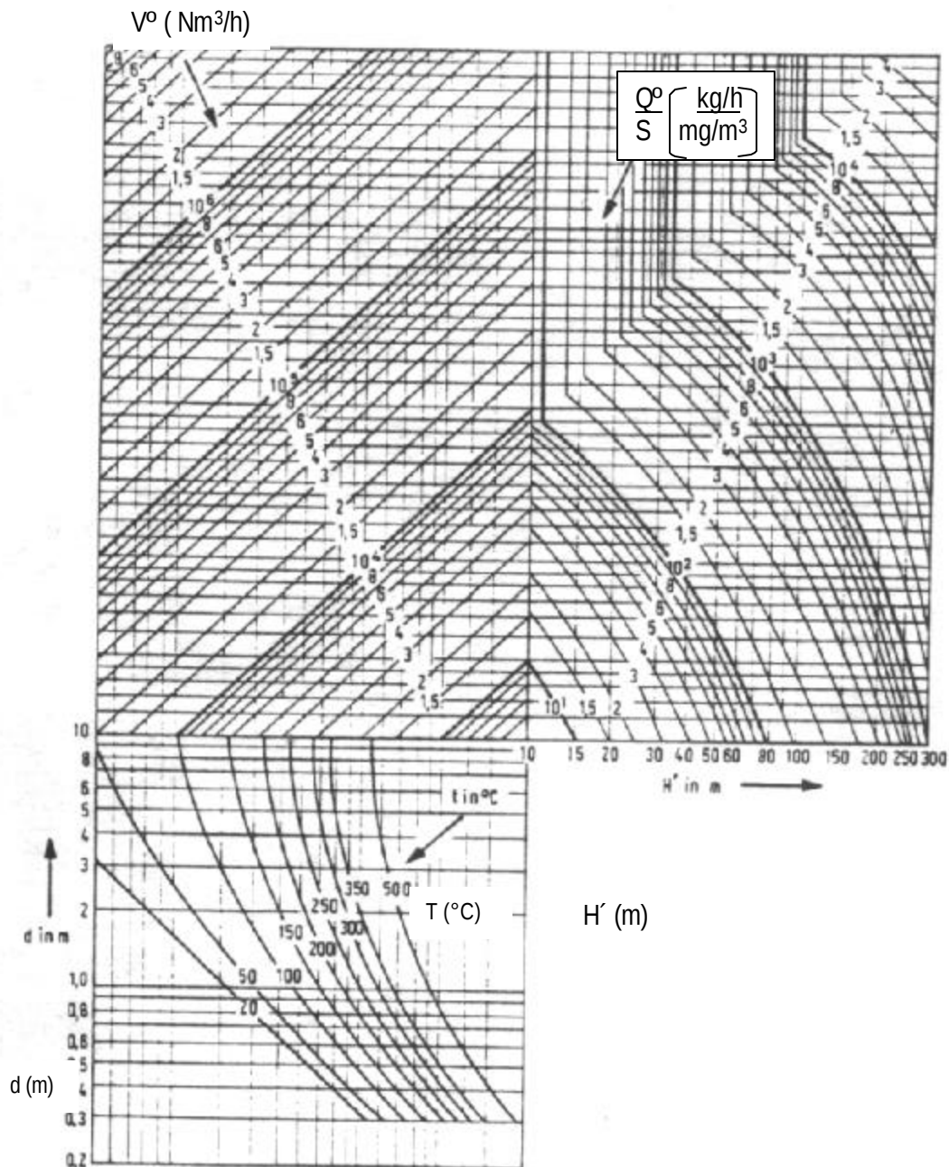
Gráfica 1. Nomograma para el calculo de la altura mínima de chimenea.
